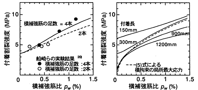
図5 横補強筋比と付着割裂強度の関係
