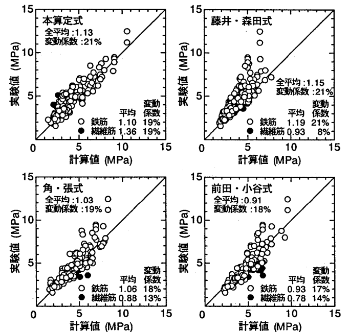
図 11 付着割裂強度の実験値と計算値の比較
