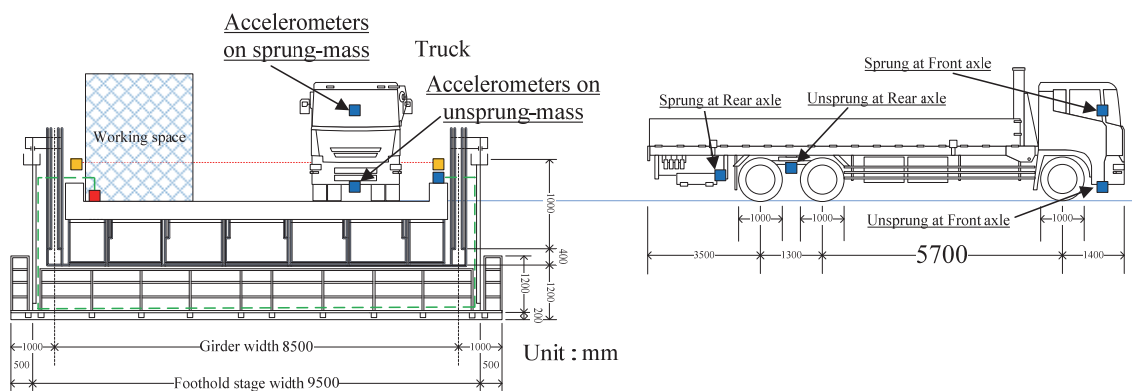
図 2.25 車両諸元
