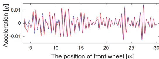
図 2.7 橋梁中央 ( x = L/2 ) の振動
