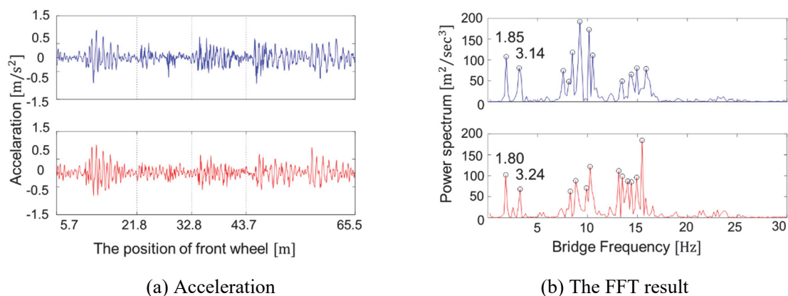
図 2.28 橋梁中点付近での加速度と FFT 結果
