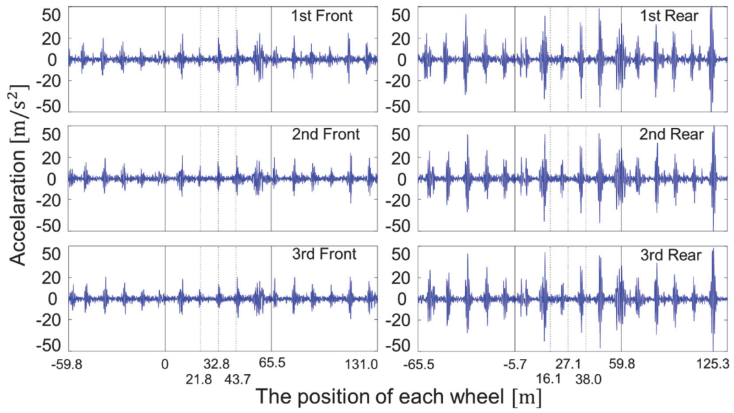
図 2.29 健全時の車両前後輪ばね下の加速度
