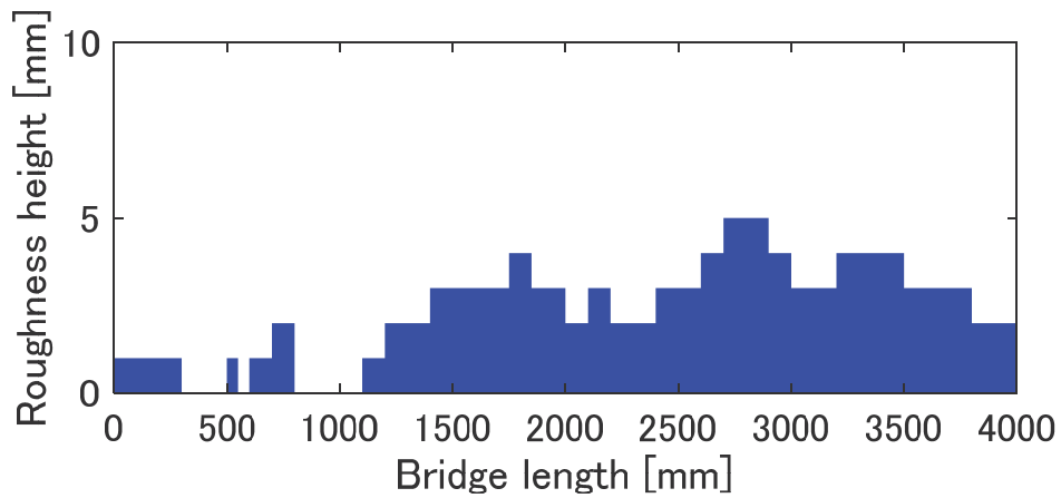
図 2.16 路面凹凸
