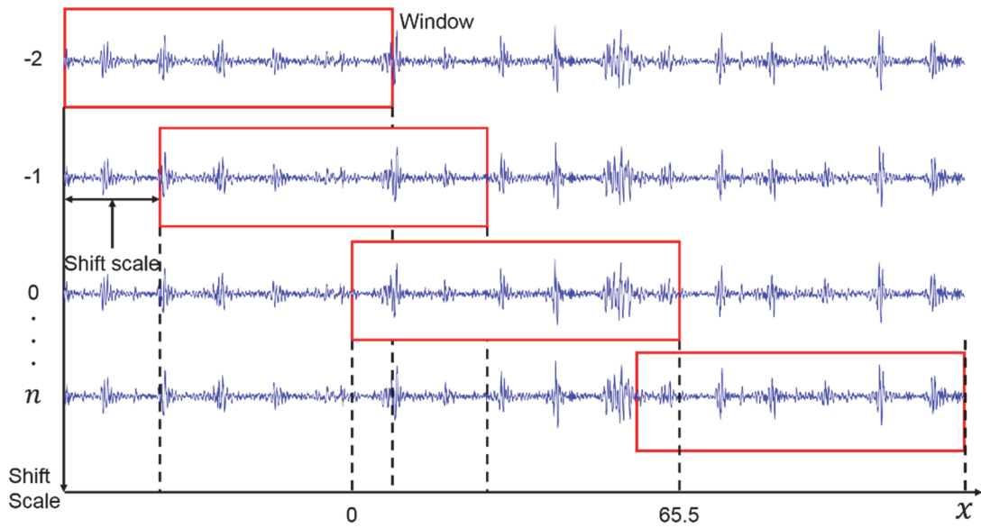
図 2.33 加速度データのシフト方法
