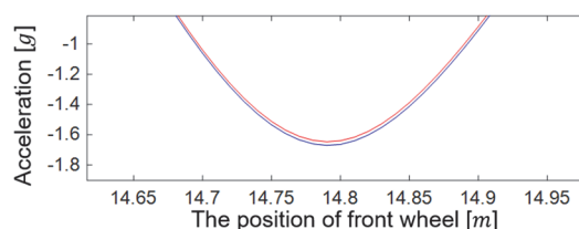
図 2.6 損傷位置でのばね下加速度 の拡大図
