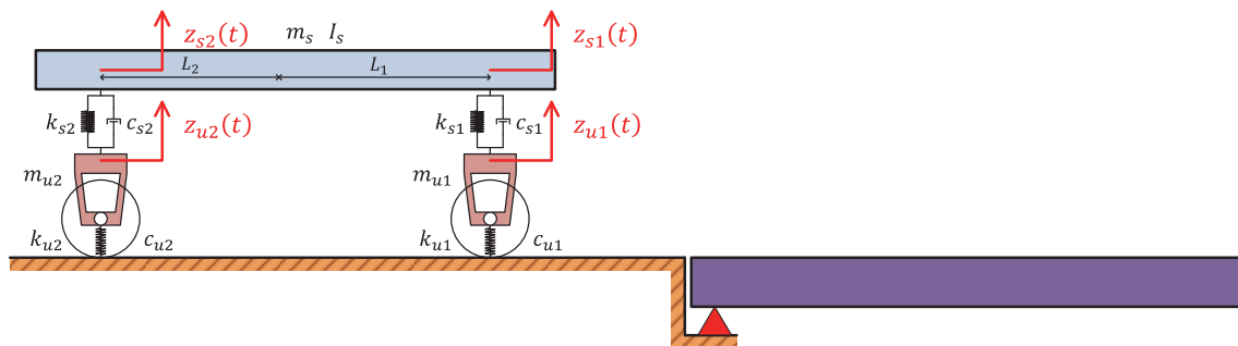
図 2.1 車両システム (Half-Car モデル)
