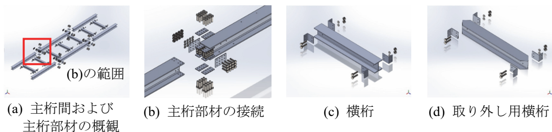
図 4.2 模型橋梁の CAD 分解図面
