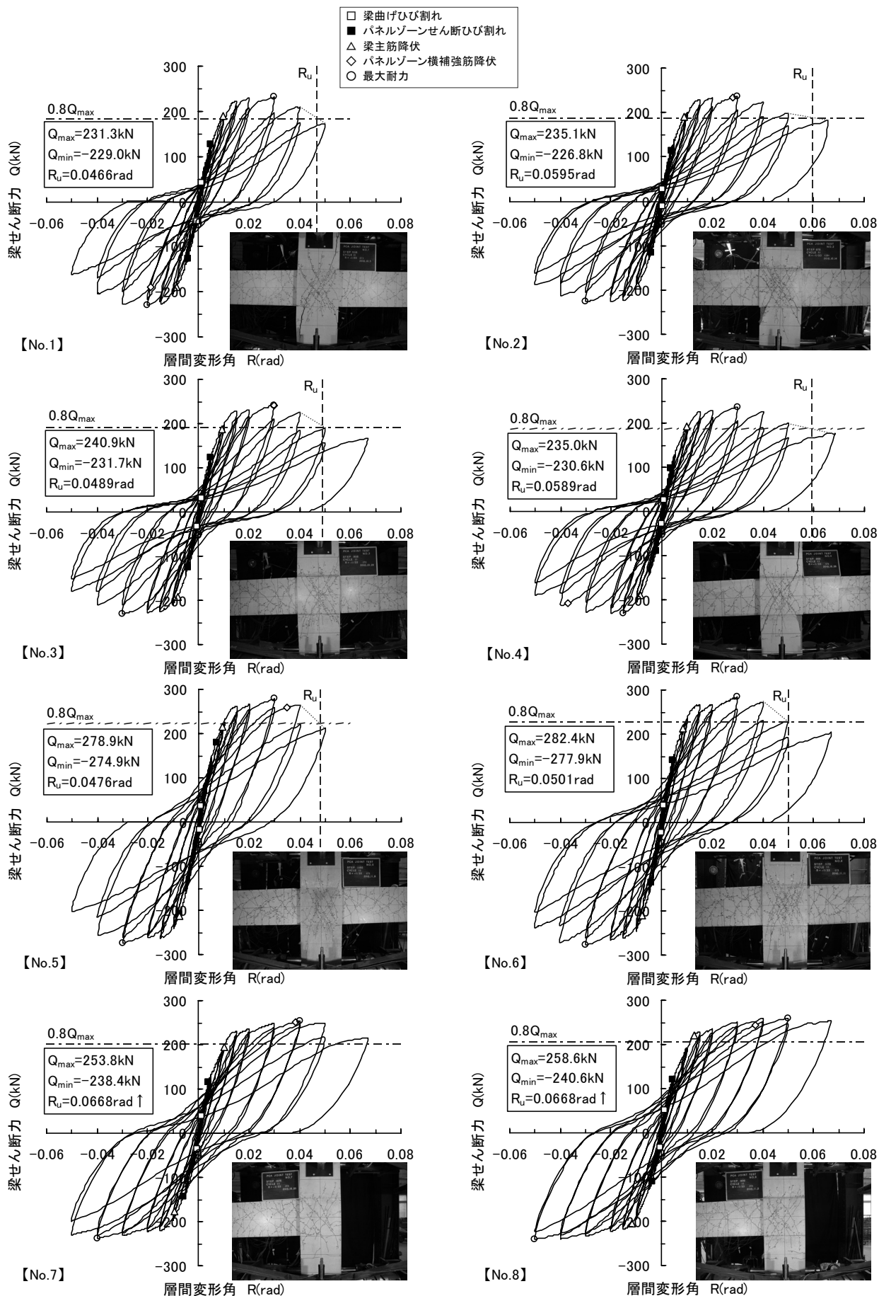
図3 梁せん断力-層間変形角曲線と破壊状況 ( R=1/33\text{rad} )
