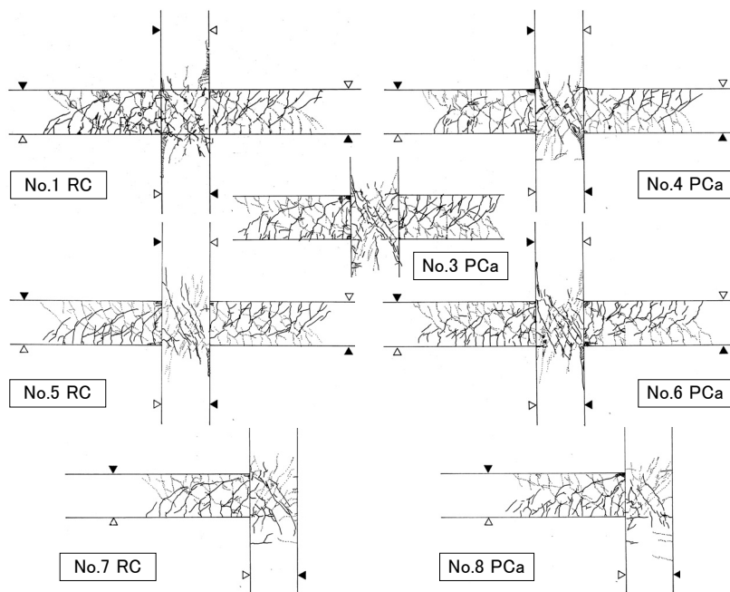
図 4 ひび割れ状況 ( R=1/33\text{rad} )
