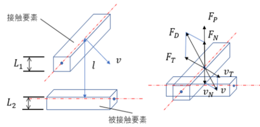
図-4 ペナルティ接触理論の概念図
